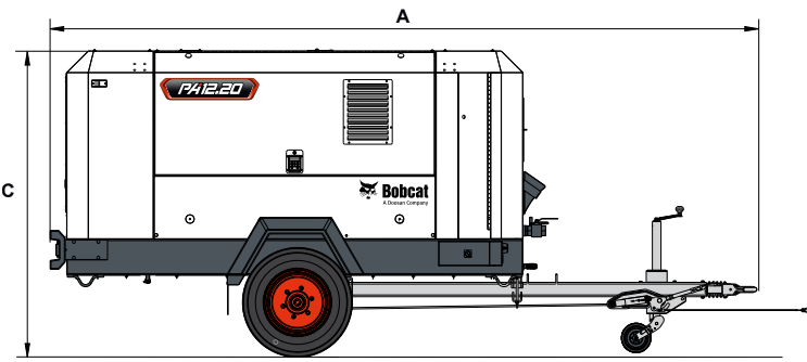
PA14.14 — loopwerk met vaste hoogte
